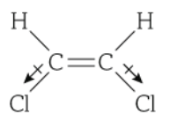
cis -dichloroethene
