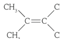
trans -2,3-dichlorobut-2-ene
