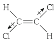
trans -dichloroethene
