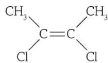
cis -2,3-dichlorobut-2-ene
